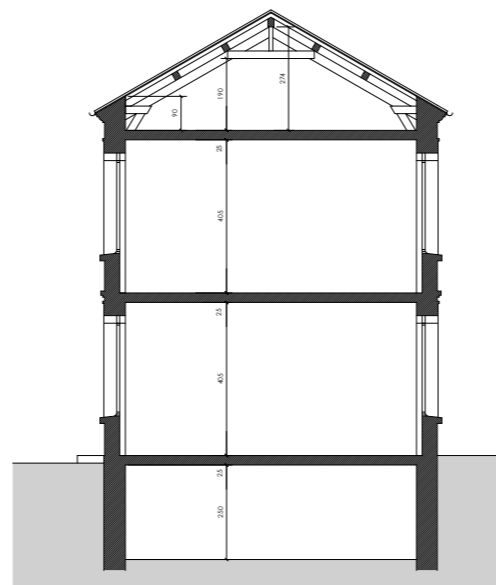
COUPE TRANSVERSALE
